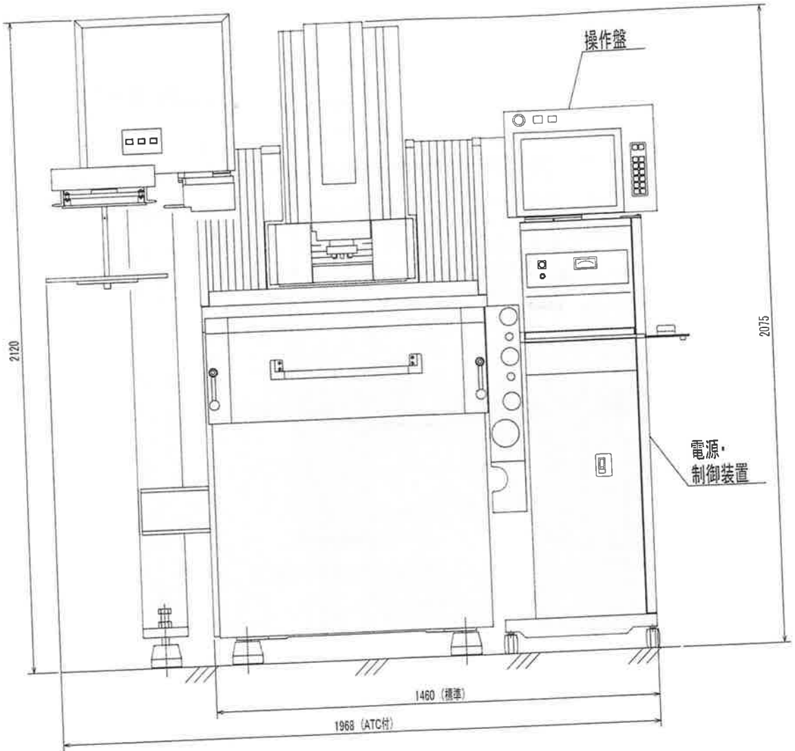
(2) EA8PVM ADVANCE 外形図
