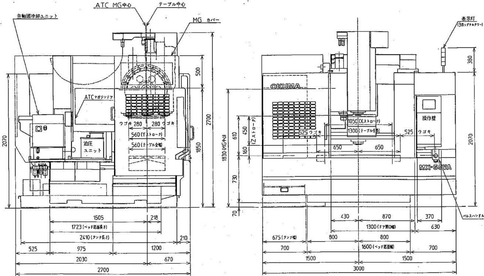
2-1. 全体寸法図 MX-55VA, MX-55VB (20本ATC)
